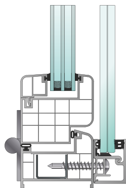
encadrement plastique et aluminium vis autoforeuse
